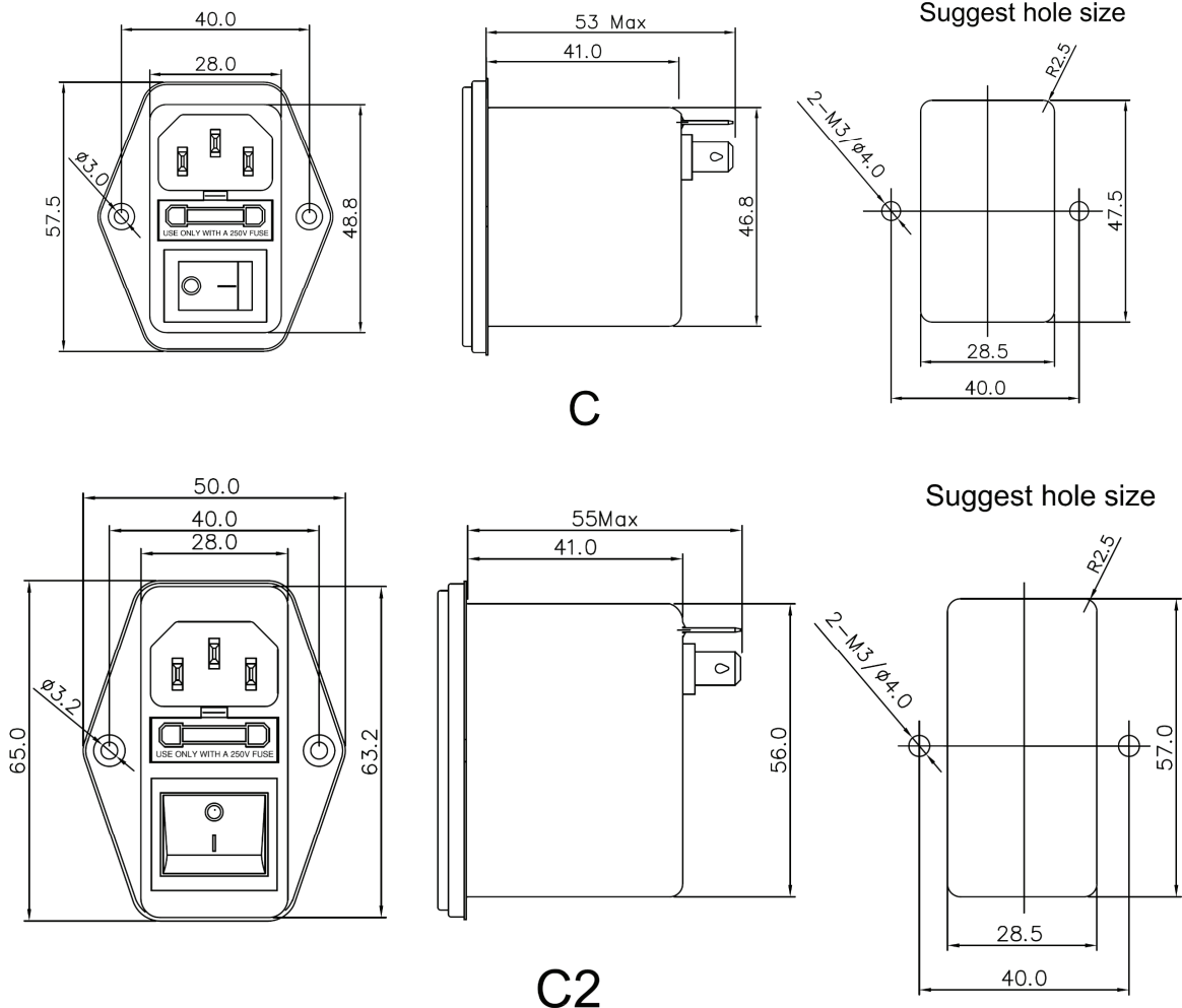
外形尺寸 Outline Dimensions(mm)
